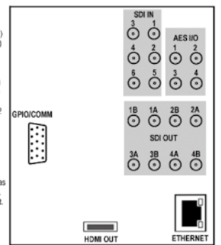
リアモジュール背面図 MPN: 1958D
