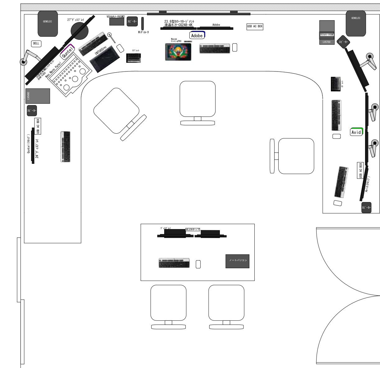
オンライン編集室配置図（第2編集室）
